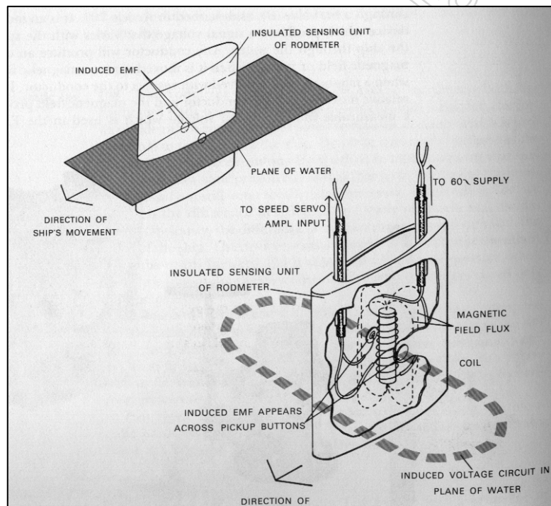
Fig. N° 4 ("Corredera Electromagnética")
