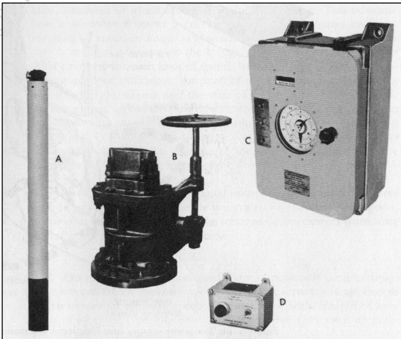
Fig. N° 3 ("Corredera Pitometer")
