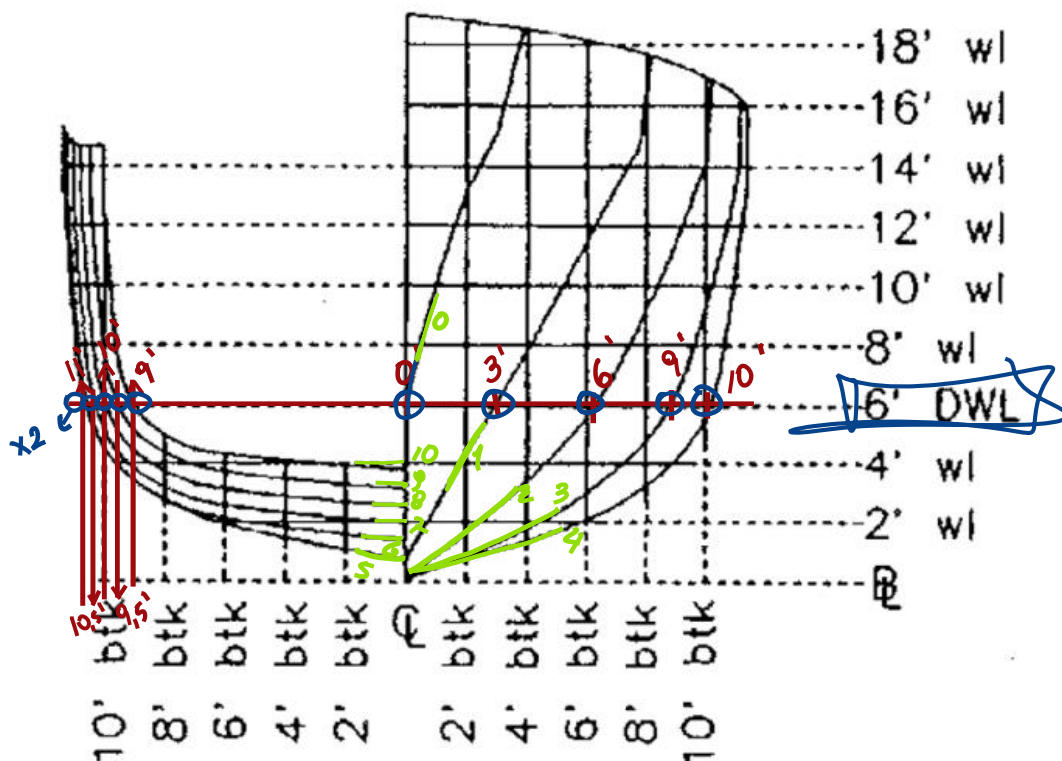
Figura 1 – Planos del Casco (Vista de frente o plano de cuerpo) del patrullero 3L
