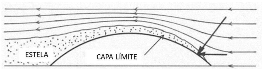
Figura 7.8 – Flujo de agua alrededor de un cuerpo sumergido
