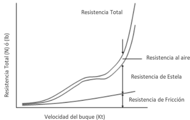
Figura 7.6 Componentes de la Resistencia del casco
