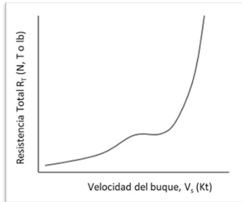
Figura 7.5 Curva típica de resistencia total del casco
