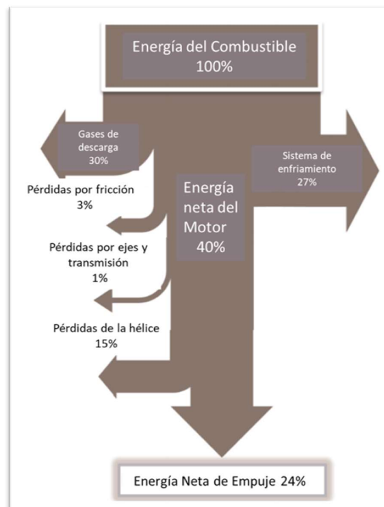
Figura 7.2 Pérdidas típicas de energía en un sistema de propulsión a bordo
