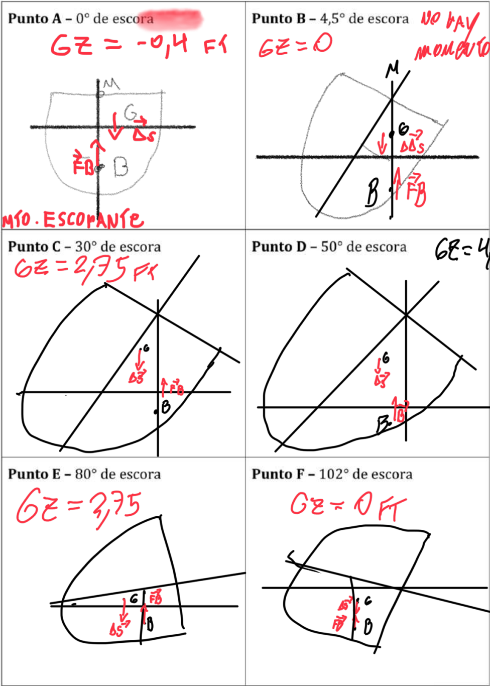
Figura 4.8 Diagramas de vectores asociados a la Figura 4.7
