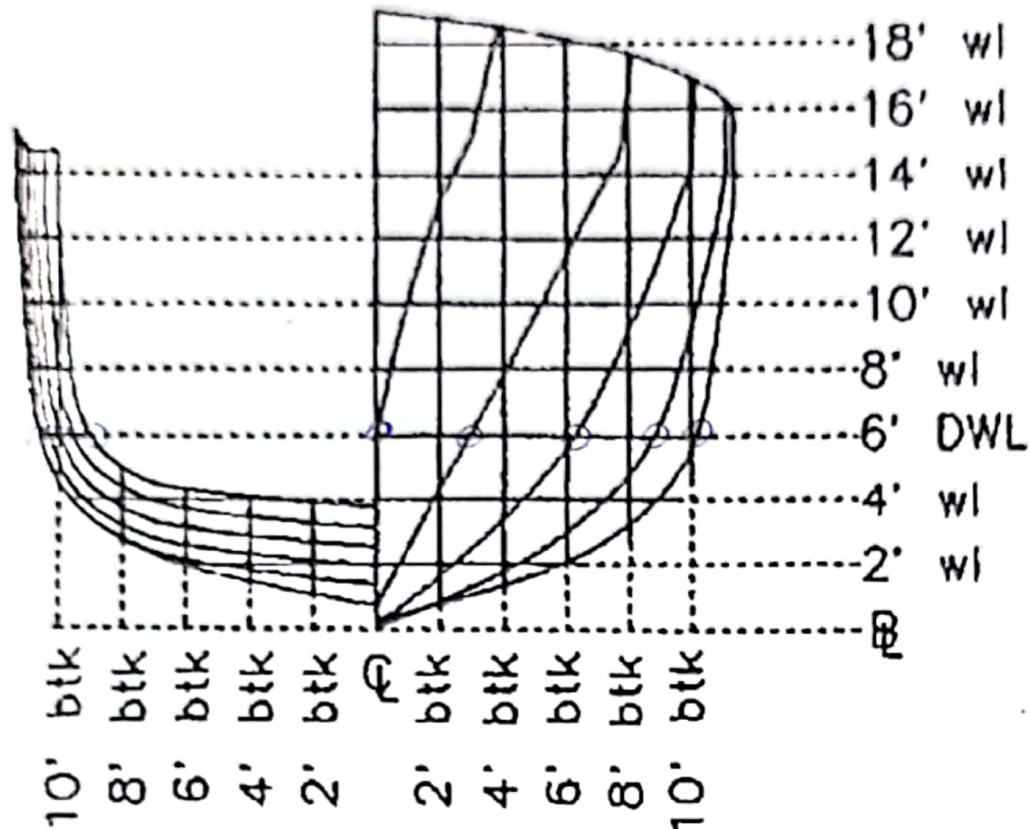
Figura 1 – Planos del Casco (Vista de frente o plano de cuerpo) del patrullero 3L
