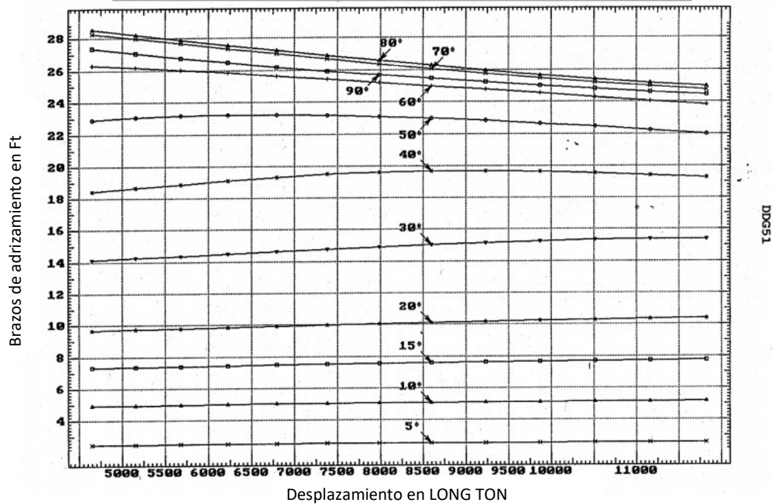
CURVAS CRUZADAS DE ESTABILIDAD – Escoras a estribor Buque inicialmente adrizado
