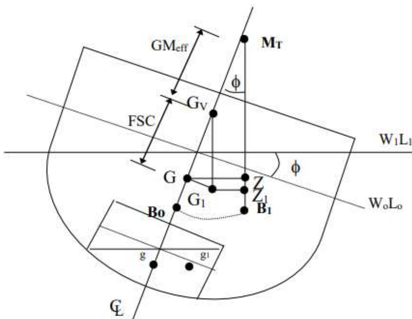
Figura 4.9 La corrección de Superficie Libre
