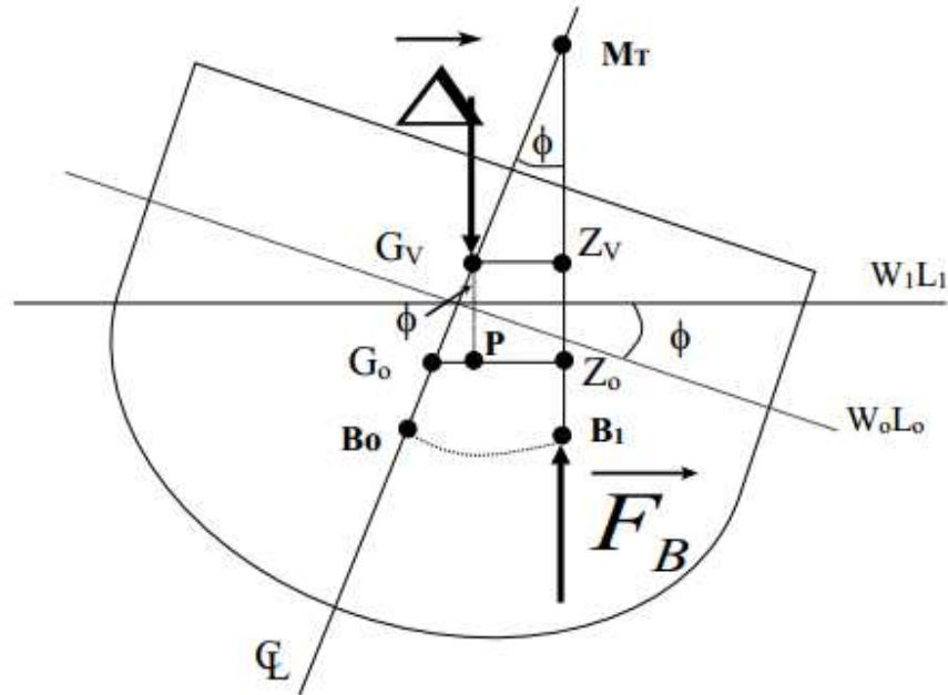
Figura 4.5 La derivación de la corrección por seno
