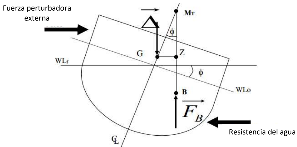
Figura 4.1 Buque escorado por un par externo
