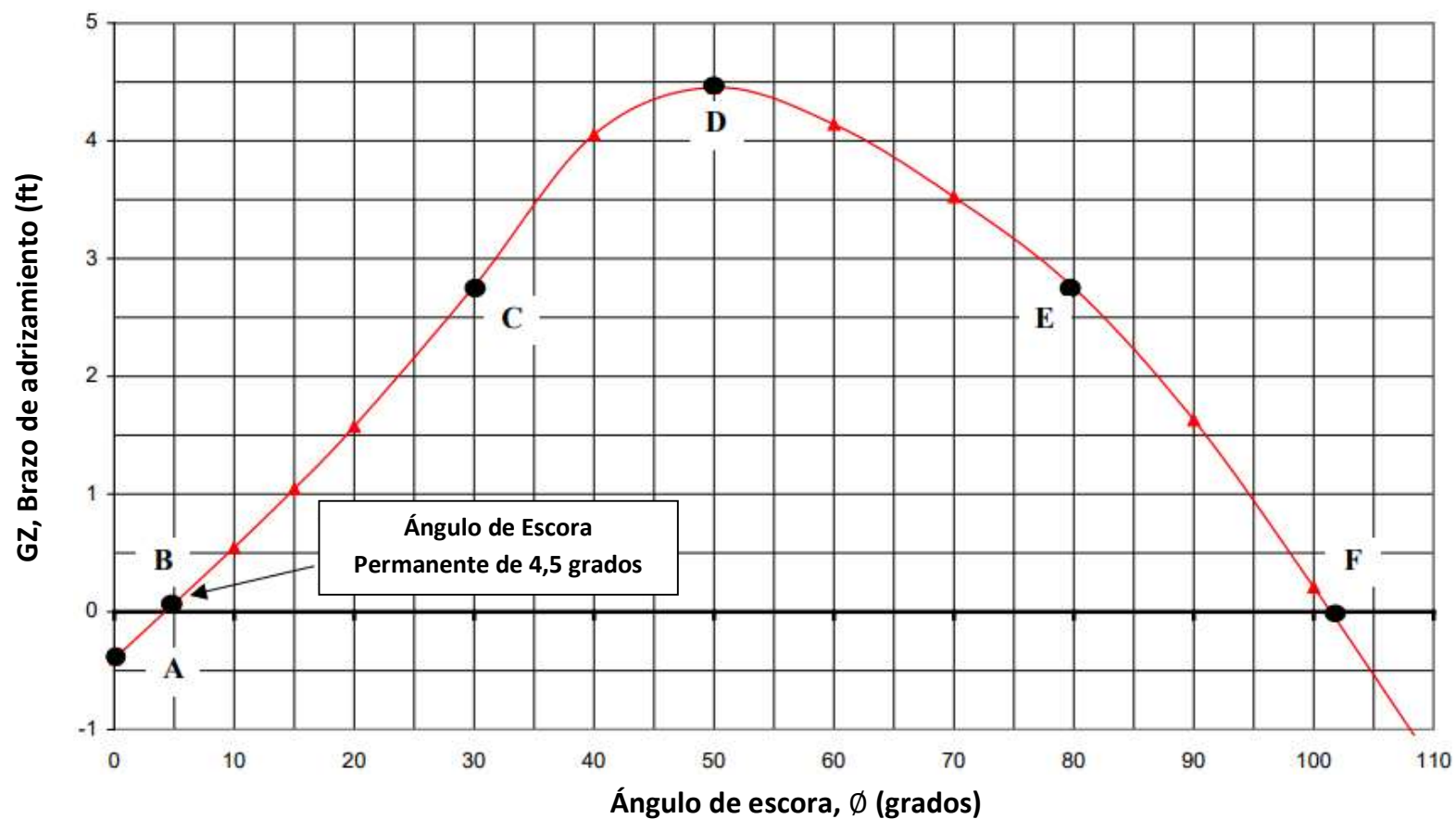
Figura 4.7 Curva de Estabilidad Estática para ejercicio del Alumno
