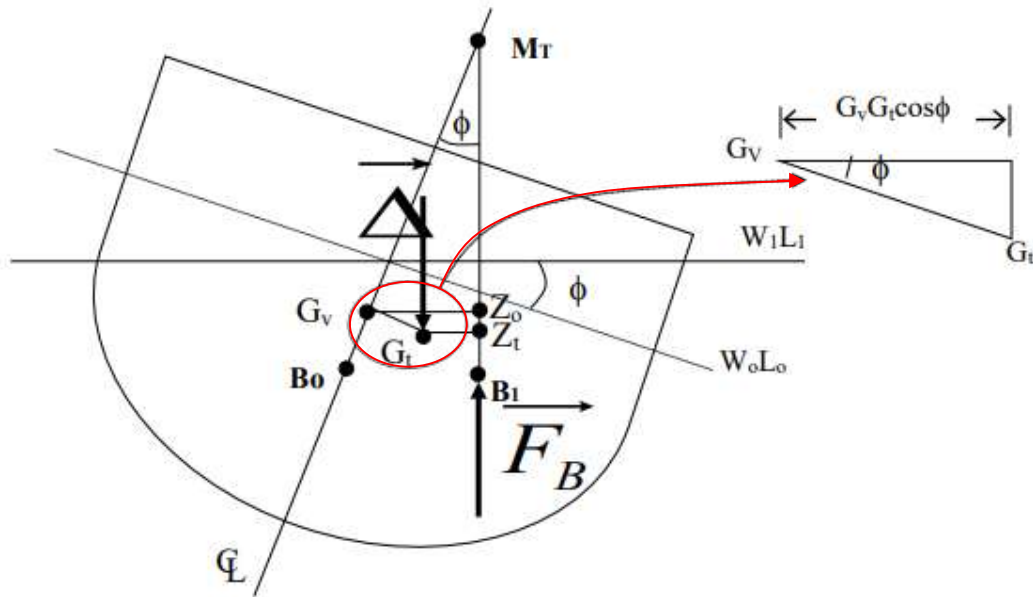
Figura 4.6 Derivación de la corrección por coseno
