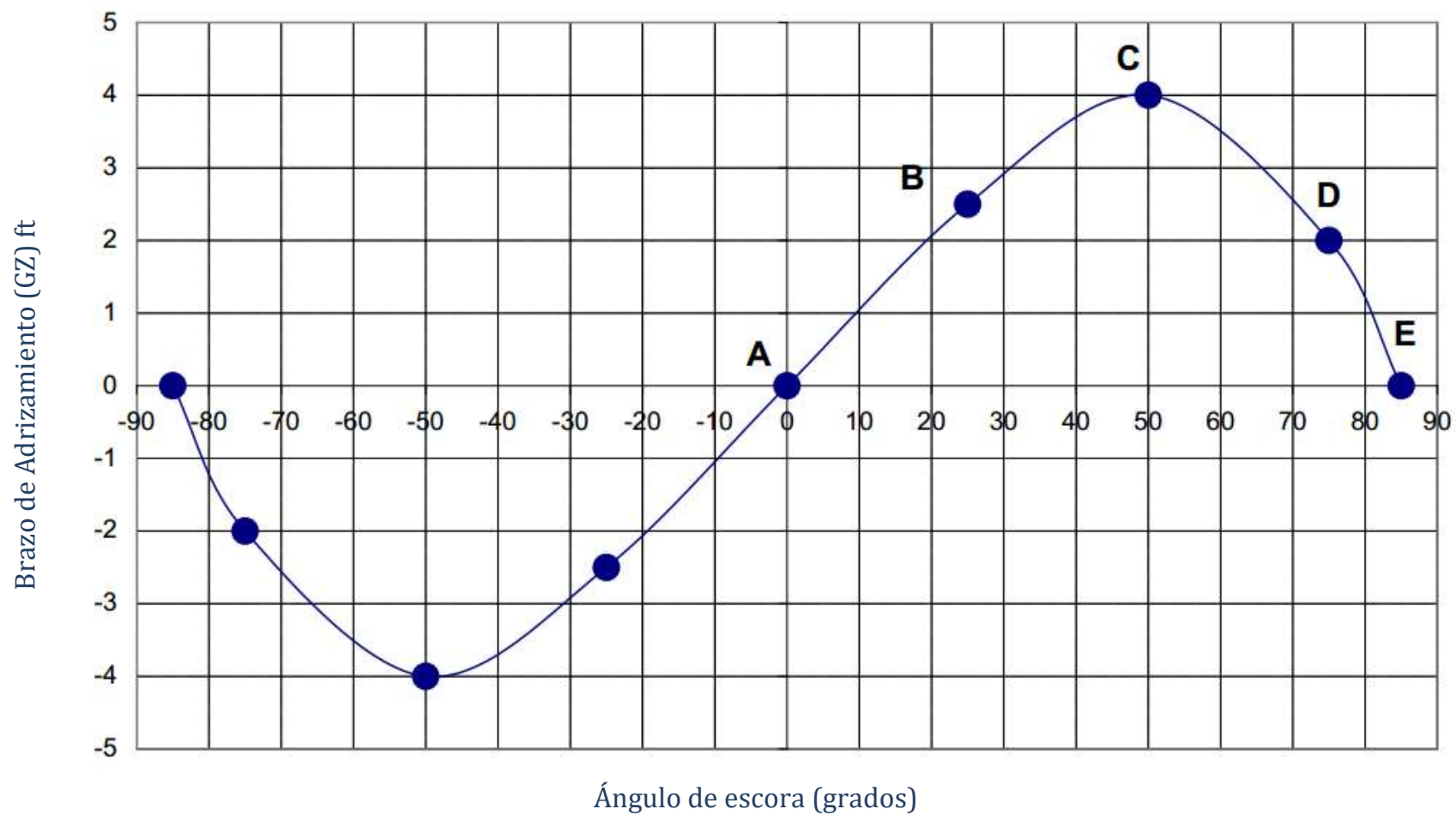
Figura 4.2 Curva de Estabilidad Estática Intacta.
