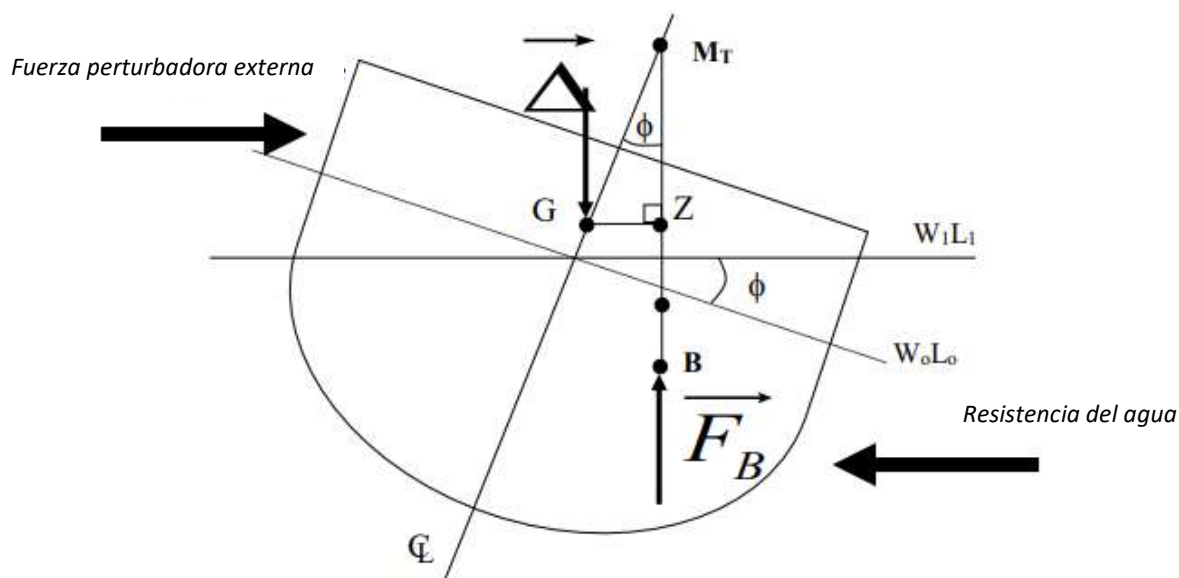
Figura 4.11 Un casco escorado a pequeños ángulos de inclinación
