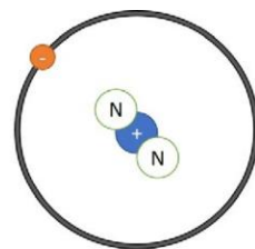
TRITIO 2 neutrones 3 masa atómica Radioactivo 0.000001 % del H terrestre
