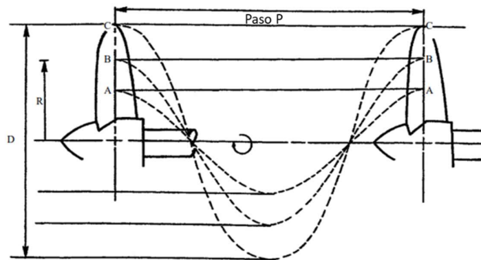
Figura 7.19 Avance de una hélice típica en una revolución. (Ref. "Introducción a la arquitectura naval" de Gillmer y Johnson)
