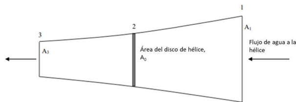
Figura 7.22 Flujo por sección transversal de área
