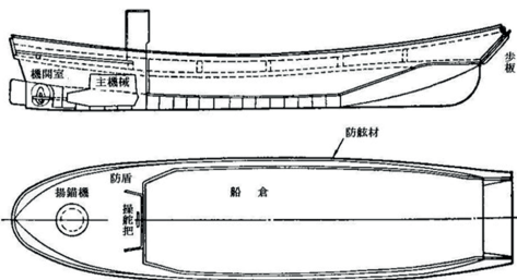
Arriba izquierda, Akitsu-Maru. Arriba derecha, Shinshū-Maru. Abajo, lanchas de desembarco japonesas Army Type "A" y "B"
