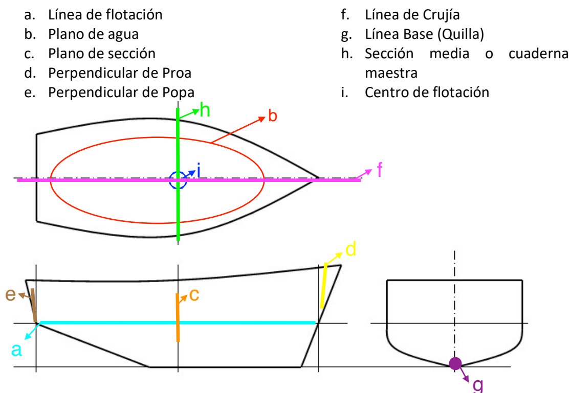
Figura 2 - Diagrama para las definiciones de forma del casco
