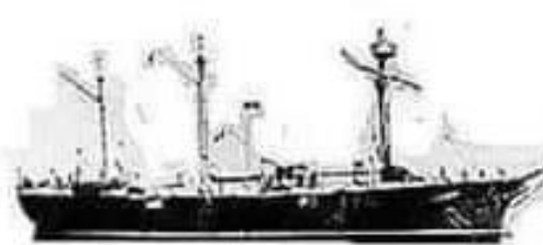
Cañonera Magallanes (1874) Desplazamiento: 950 Toneladas Art. Principal: 1 Cañón de 115 lb Blindaje: Casco madera Velocidad Max: 11,5 Nudos
