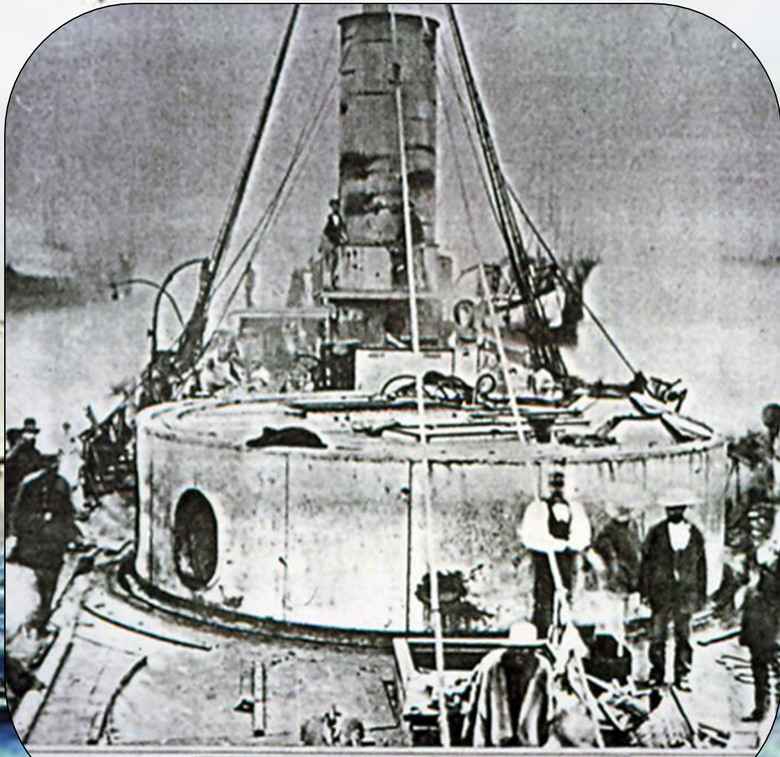
DESTRUCTOR HUASCAR ▲ FAENA DE AGUA EN HUASCO - AÑO 1879 ▲
