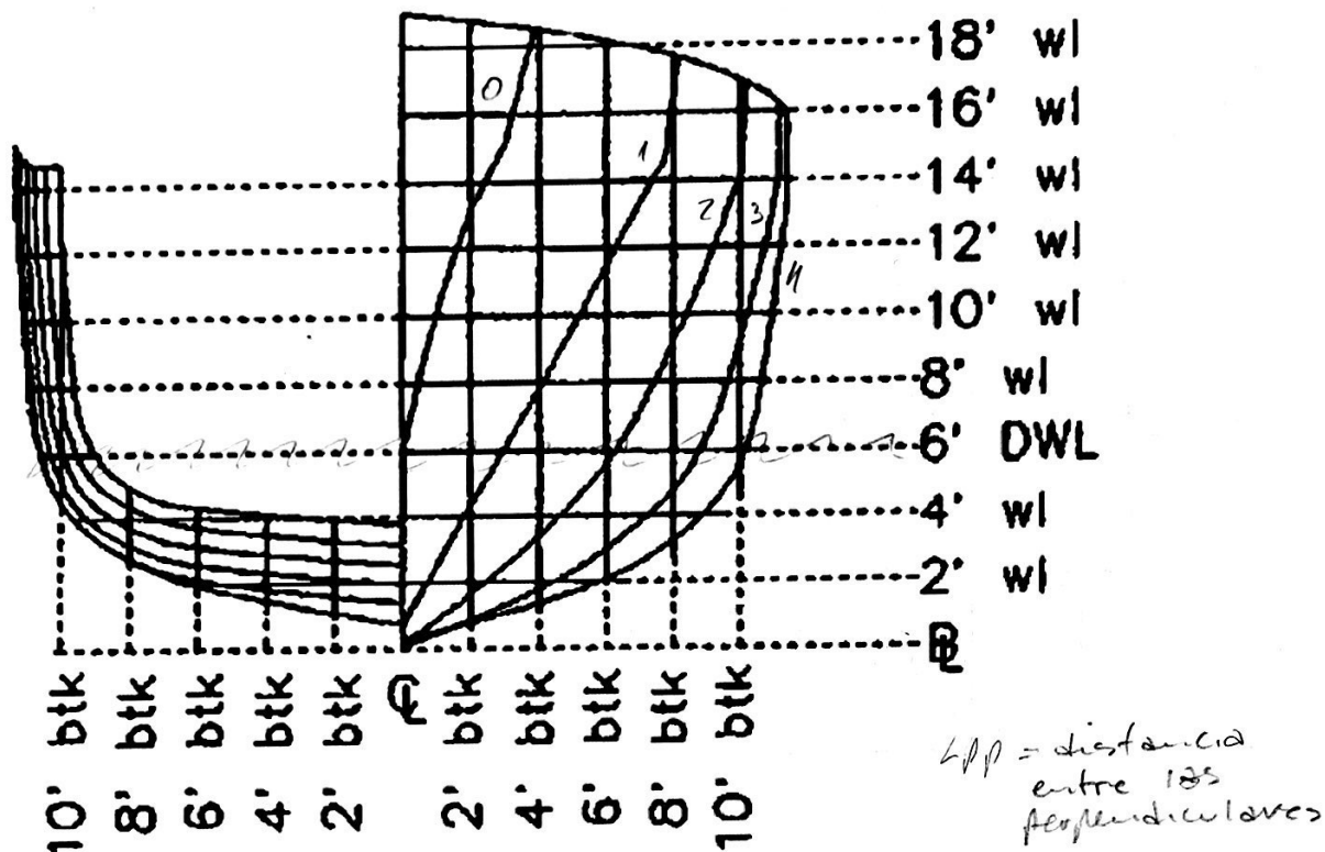
Figura 1 – Planos del Casco (Vista de frente o plano de cuerpo) del patrullero 3L
