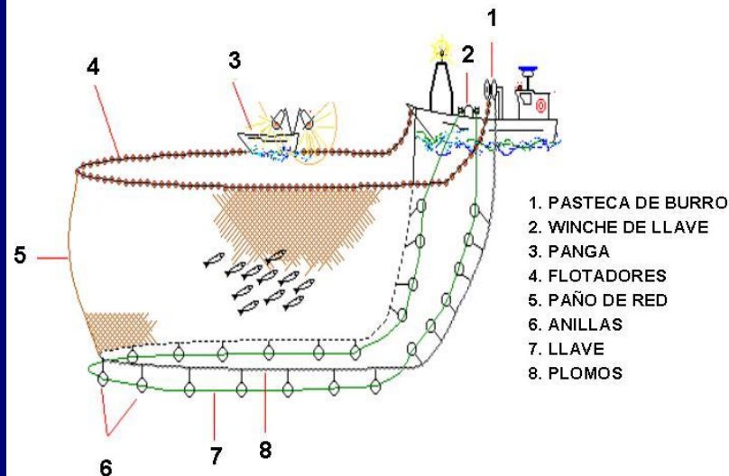
ESQUEMA GENERAL DE UN ARTE DE PESCA DE CERCO
